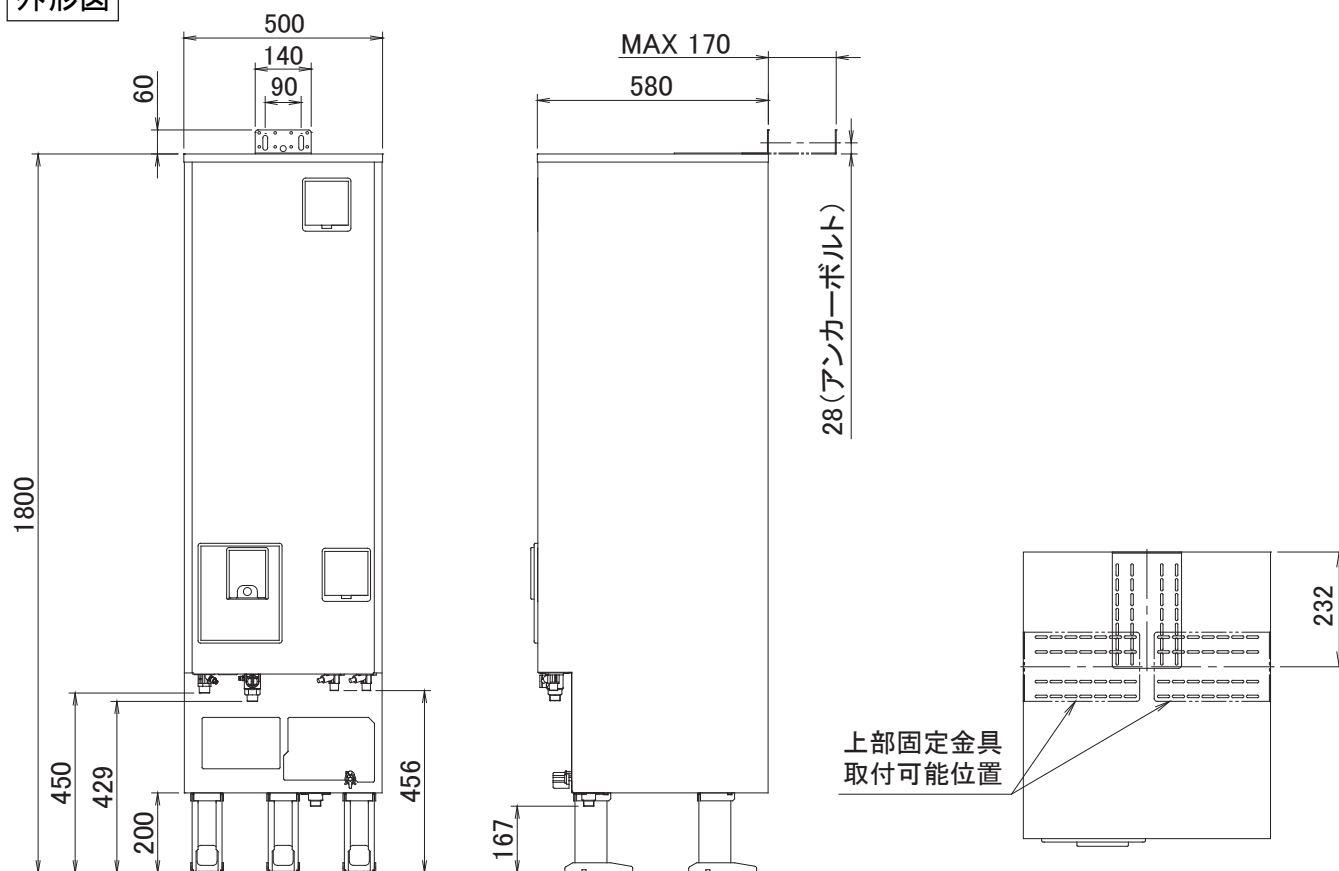
外形圖
