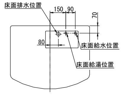
ボウルセンター
