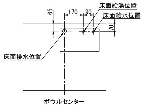
アクリル人大フラットカウンター 2段スライドタイプ間口75cm ヘルスマーター収納タイプ間口75cm
