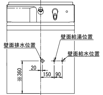
ホーローボウル壁出水栓
