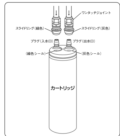
●カートリッジ部・拡大図
