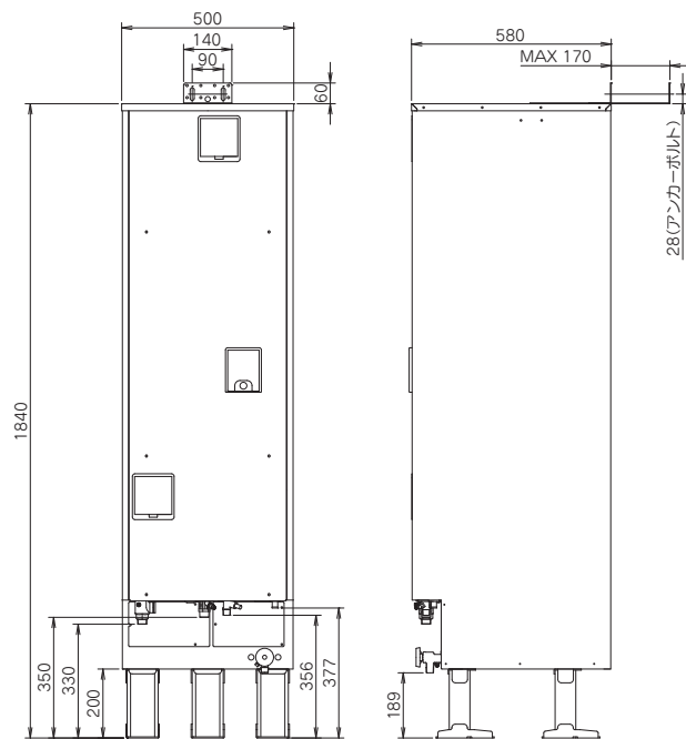
《外形図》
