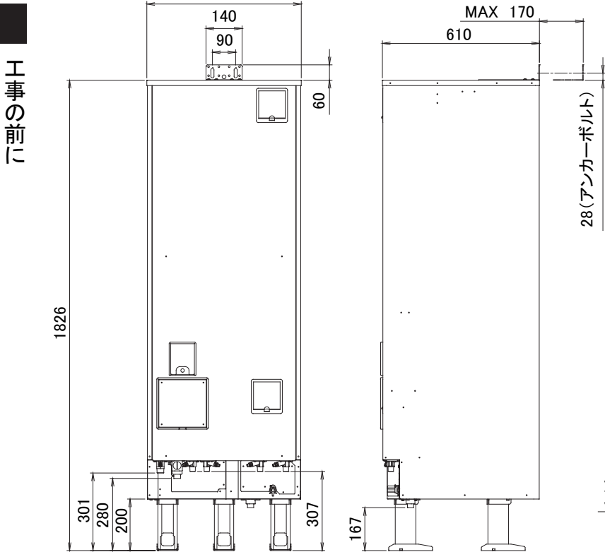
《外形図》
