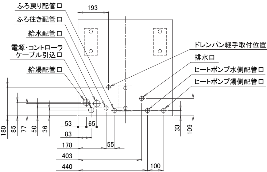
《配管位置図》
