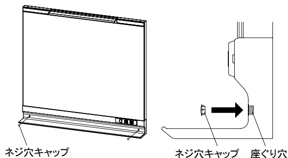
側面図
