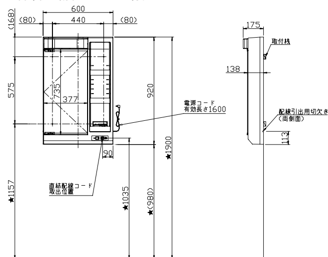
SIM-060M1AHY/(N)E タイプ
