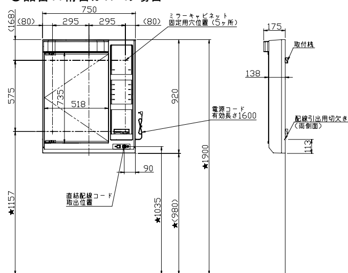
SIM-075M1AHY/(N)E タイプ
