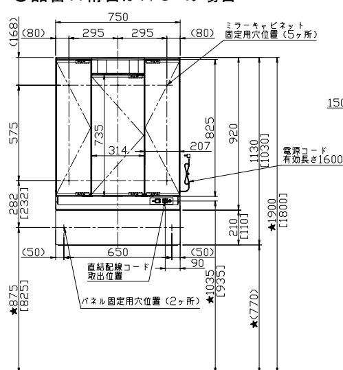
SIM-075M3AFY/(N)E タイプ SIM-075M3ASY/(N)E タイプ SIM-075M3DFY/(N)E タイプ SIM-075M3DSY/(N)E タイプ
