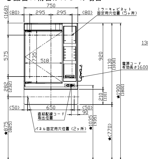
SIM-075M1AFY/(N)E タイプ SIM-075M1ASY/(N)E タイプ
