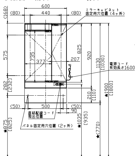
SIM-060M2AFY/(N)E タイプ SIM-060M2ASY/(N)E タイプ
