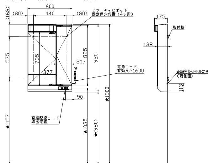
SIM-060M2AHY/(N)E タイプ
