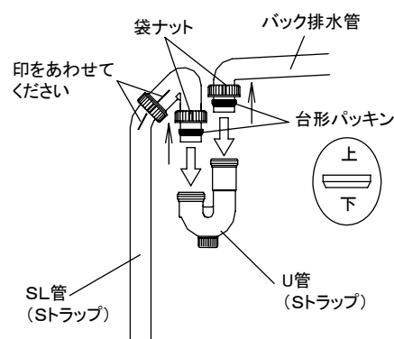
床排水の場合
