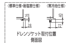
側面図
