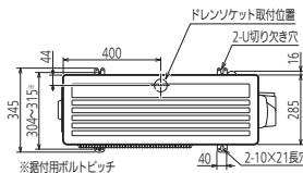
上面図
