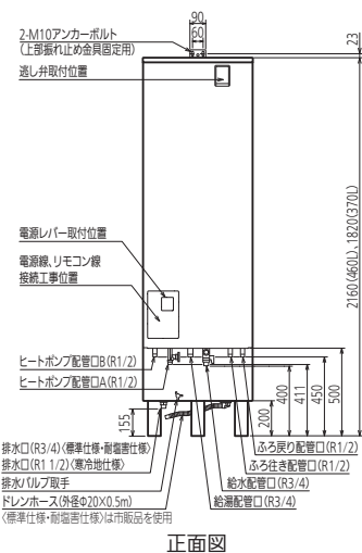
正面図
