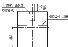
上面図
