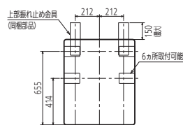
上面図
