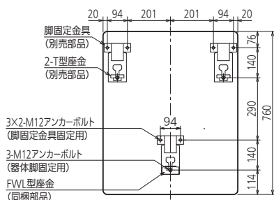
アンカーボルト位置(上面透視図)
