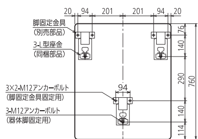
アンカーボルト位置(上面透視図)
