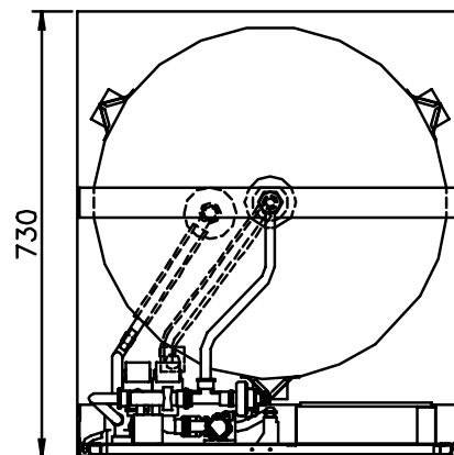
上面透視図
