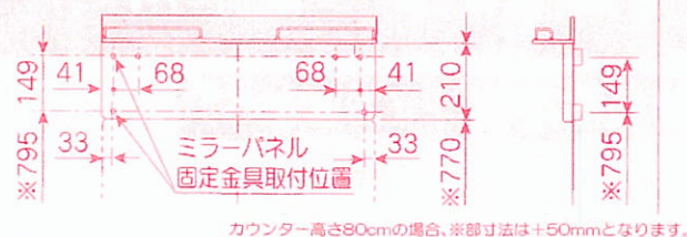
ミラーパネル取付寸法位置 (間口75cmオンディース、薄型タイプの場合)
