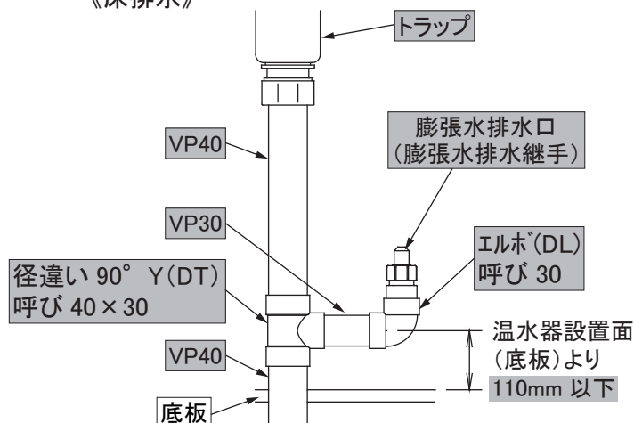
膨張水排水継手 (現地作製)
