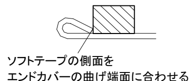
ソフトテープ 貼付部断面図
