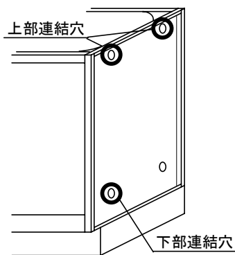
＜シンク・調理キャビネットとの連結＞
