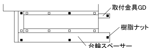
天板高さ900mmの場合
