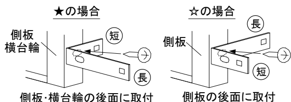
取付金具GD 取付部
