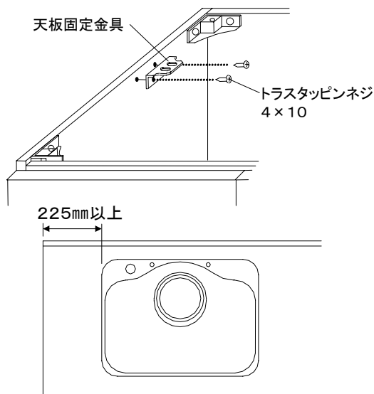
＜シンクがセットエンド側に寄っていない場合＞
