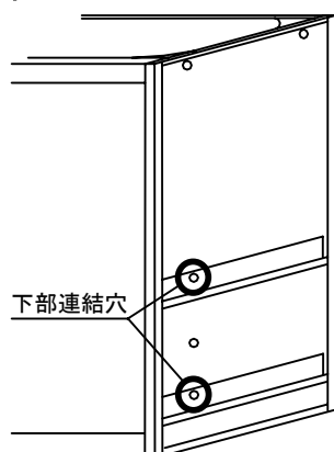
＜コンロキャビネットとの連結＞
