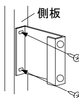
△取付金具GUZ 取付部
