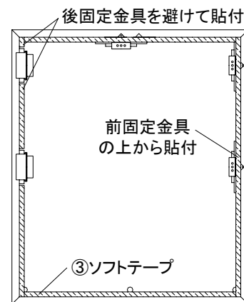
ソフトテープ 貼付部断面図
