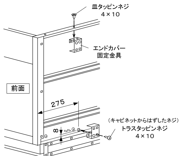
<取付金具DV>
