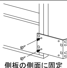
▲取付金具GUY 取付部
