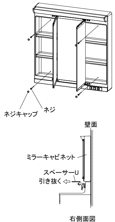
右側面図
