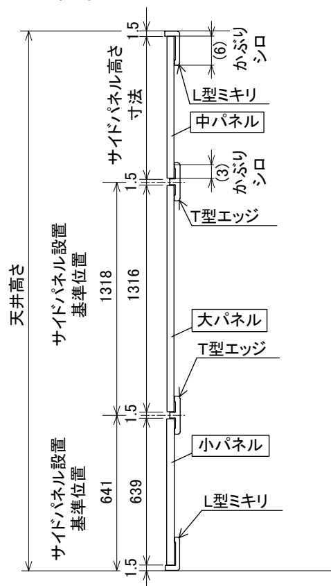
◎サイドパネル 標準割付図(正面図)
