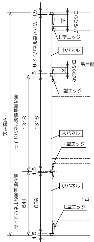
◎サイドパネル 標準割付図（正面図）
