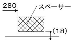
◇ スペーサー 貼付部
