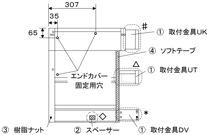
天板高さ900 の場合
