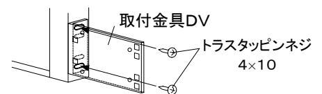
* 取付金具DV 取付部
