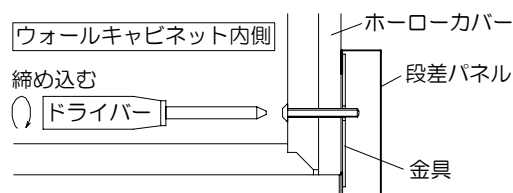
段差パネル取付図
