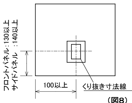
コンセント取付穴寸法図
