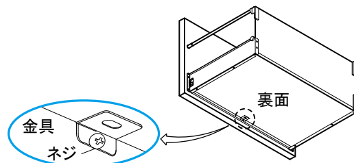
＜取付方法＞
