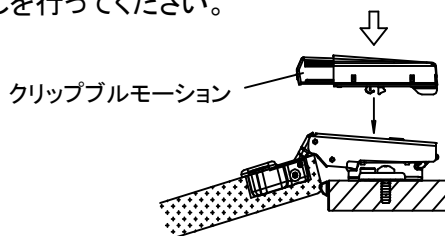
＜取付方法＞
