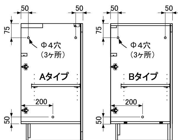
<連結用下穴位置>
