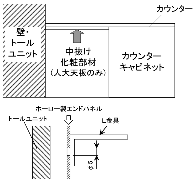
L金具をエンドパネルに取り付けた場合の断面図
