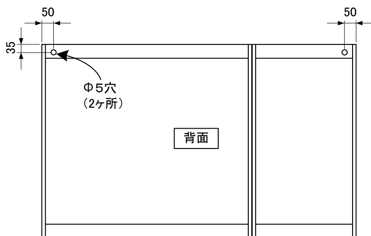
<壁面固定用下穴位置>
