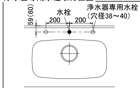
浄水器専用水栓取付位置
