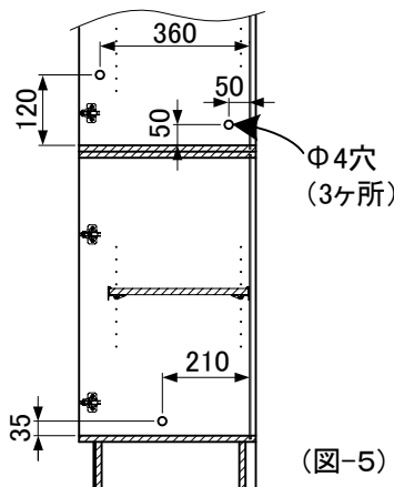
<ツールユニットへの連結用下穴位置>
