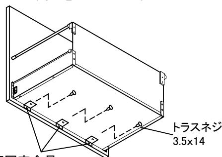
前板固定金具
