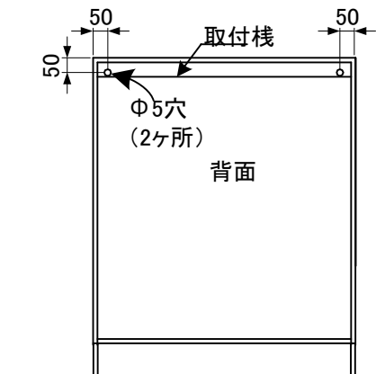
(図-4) <壁面固定用下穴位置>
