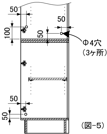
(図-5) <ツールユニットとの連結用下穴位置>
