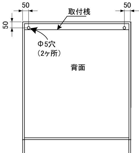
＜壁面固定用下穴位置＞ (図-4)
