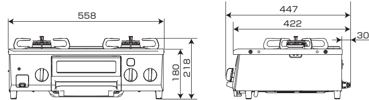
■外形寸法図（単位：mm）
