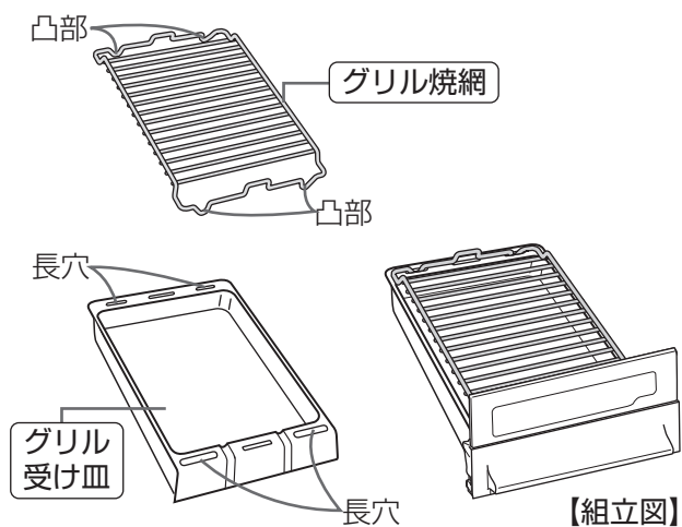
焼物を高い位置で焼く場合
