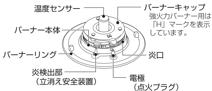
強火力バーナー・標準バーナー
