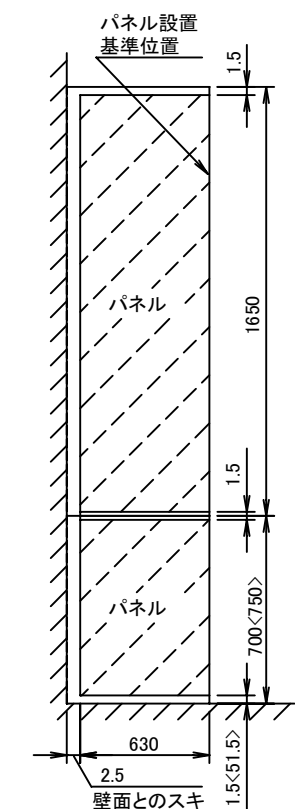
高さ235cmタイプ PSP-YDHHA
