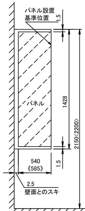
カンタン取付タイプ PSP-YMSLA・YDSL A
