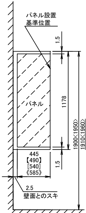
カンタン取付タイプ PSP-YSA・YMSA・YCSA・YDSA
