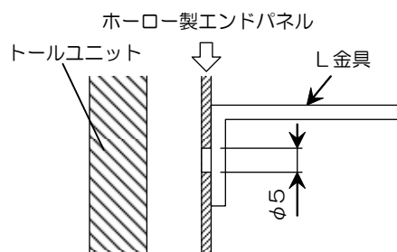
L金具をエンドパネルに取り付けた場合の断面図
