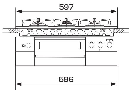
トッププレート巾 60cmタイプ
