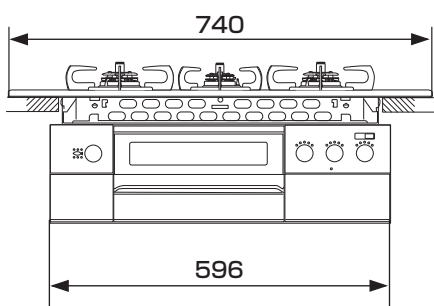
トッププレート巾 75cmタイプ
