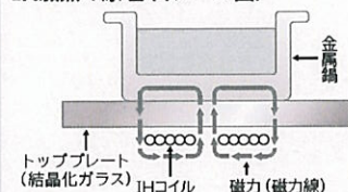
IH加熱の原理(イメージ図)
